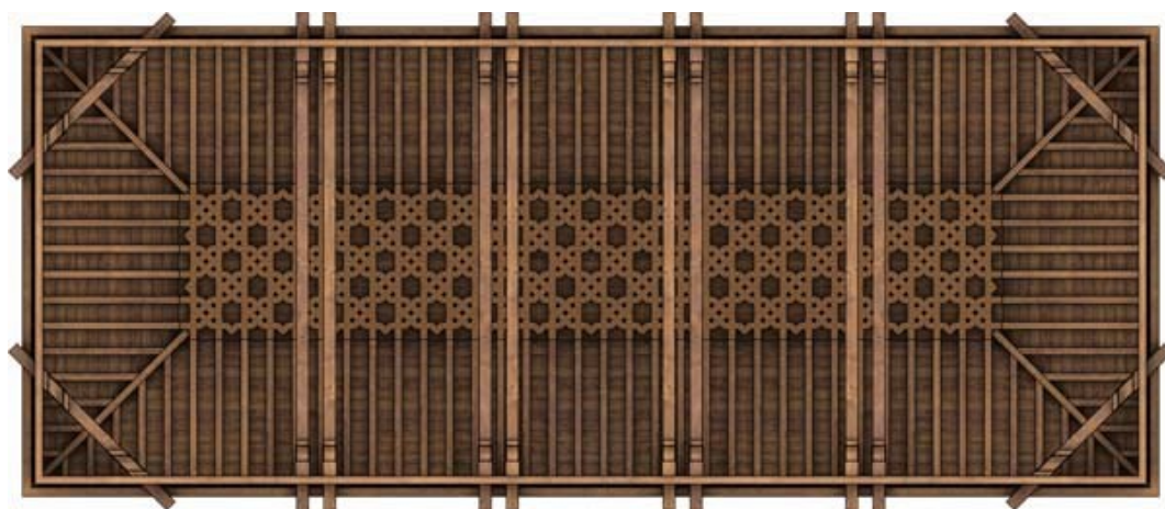
Armadura mudéjar de la nave central
